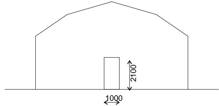
julkisivu oikealta
